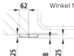
Winkel flucht
