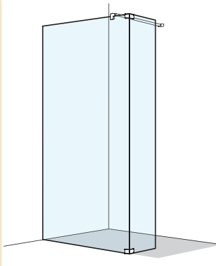
Walk-In Trennwand m. Fixelement 2-teilig, J-WIF
